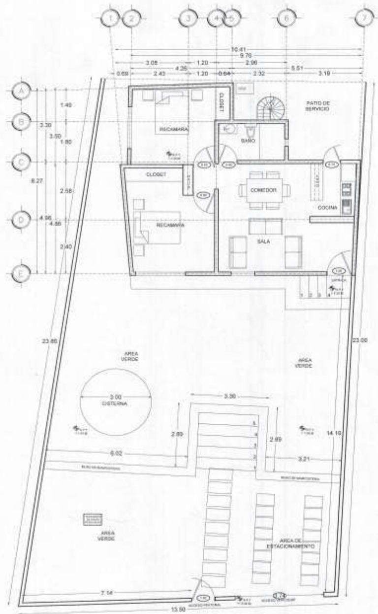
PLANTA ARQUITECTONICA CASA HABITACION CONSTRUCION BL 7115 AREA DE CONSTRUCCION EN SUFIA, 14.10 M 2 PLANTANIA MENDAS A LOTE
