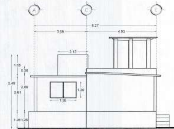
FACHADA LATERAL
